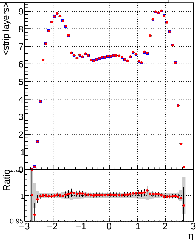
DQM_CKF_XiMinusPU_base DQM_CKF_XiMinusPU_retrainOldFiles125_v2_prelimWPM_epoch4
