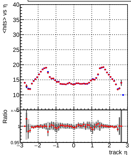
— DQM_CKF_XiMinusPU_base — DQM_CKF_XiMinusPU_retrainOldFiles125_v2_prelimWPM_epoch4
