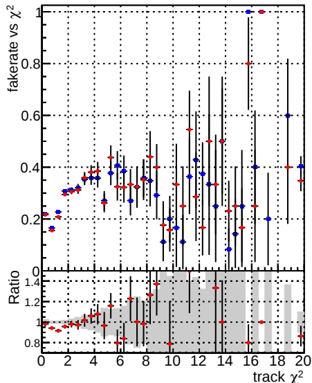
Fake rate vs. —◆— DQM CKF_XiMinusPU_base —◆— DQM CKF_XiMinusPU_retrainOldFiles125_v2_prelimWPM_epoch4
