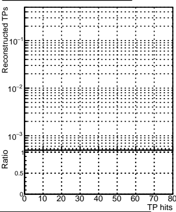
■ DQM_CKF_XiMinusPU_base ■ DQM_CKF_XiMinusPU_retrainOldFiles125_v2_prelimWPM_epoch4
