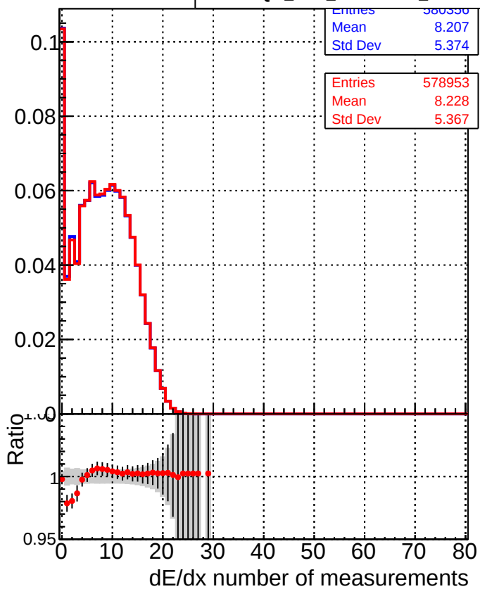
■ DQM_CKF_XiMinusPU_base ● DQM_CKF_XiMinusPU_retrainOldFiles125_v2_prelimWPM_epoch4
