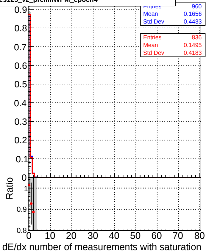
■ DQM_CKF_XiMinusPU_base ● DQM_CKF_XiMinusPU_retrainOldFiles125_v2_prelimWPM_epoch4
