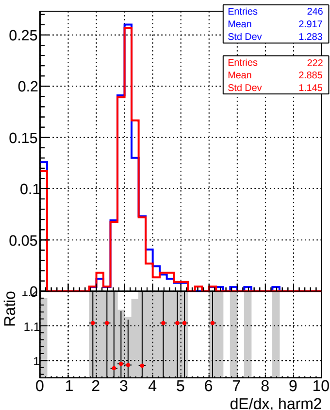
■ DQM_CKF_XiMinusPU_base ● DQM_CKF_XiMinusPU_retrainOldFiles125_v2_prelimWPM_epoch4
