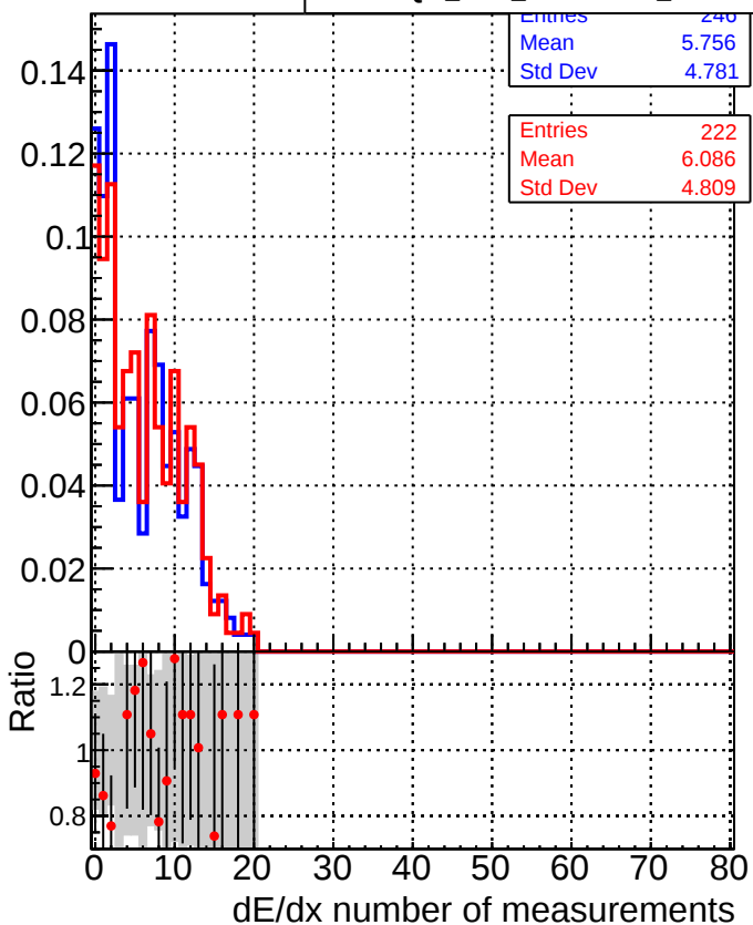
■ DQM_CKF_XiMinusPU_base ● DQM_CKF_XiMinusPU_retrainOldFiles125_v2_prelimWPM_epoch4
