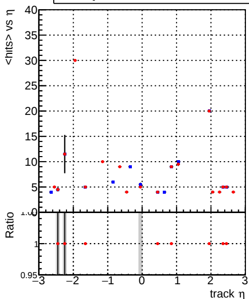
— DQM_CKF_XiMinusPU_base — DQM_CKF_XiMinusPU_retrainOldFiles125_v2_prelimWPM_epoch4
