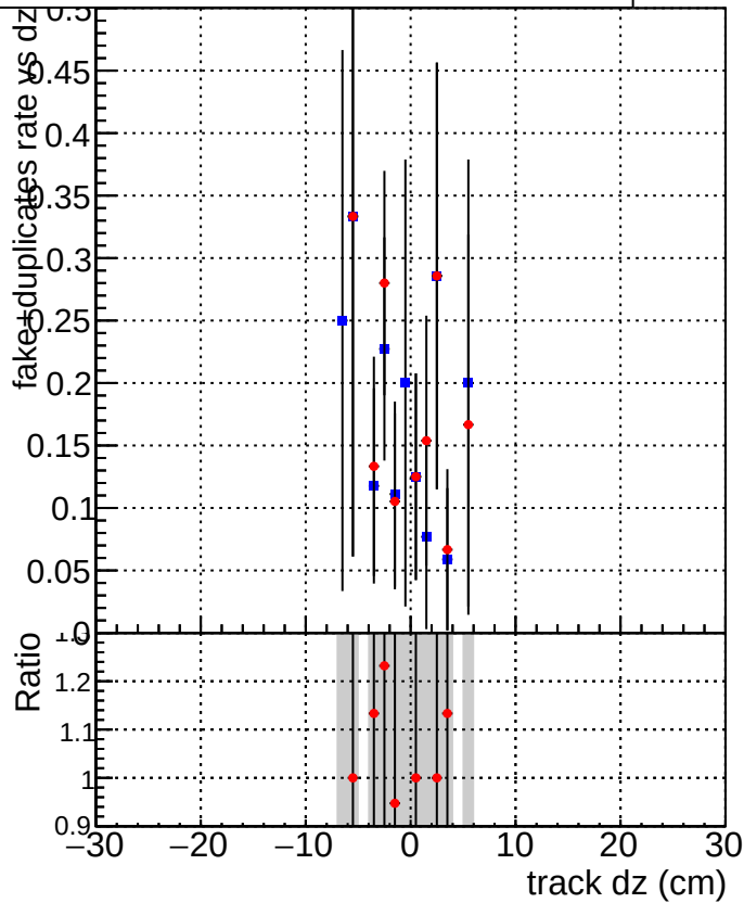
DQM_CKF_XiMinusPU_base DQM_CKF_XiMinusPU_retrainOldFiles125_v2_prelimWPM_epoch4
