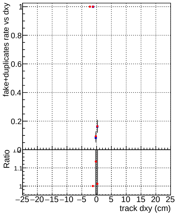
DQM_CKF_XiMinusPU_base DQM_CKF_XiMinusPU_retrainOldFiles125_v2_prelimWPM_epoch4
