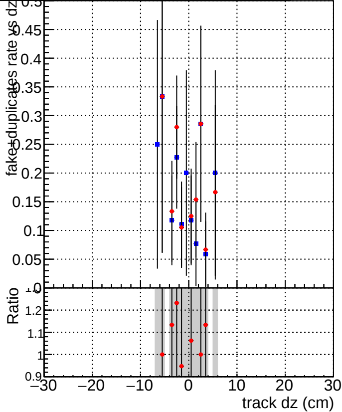
DQM_CKF_XiMinusPU_base DQM_CKF_XiMinusPU_retrainOldFiles125_v2_prelimWPM_epoch4
