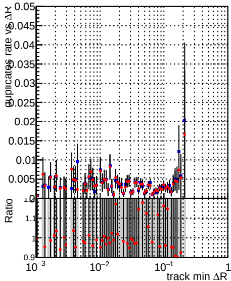
—●— DQM_CKF_XiMinusPU_base —●— DQM_CKF_XiMinusPU_retrainOldFiles125_v2_prelimWPM_epoch4
