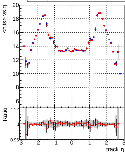
— DQM_CKF_XiMinusPU_base — DQM_CKF_XiMinusPU_retrainOldFiles125_v2_prelimWPM_epoch4
