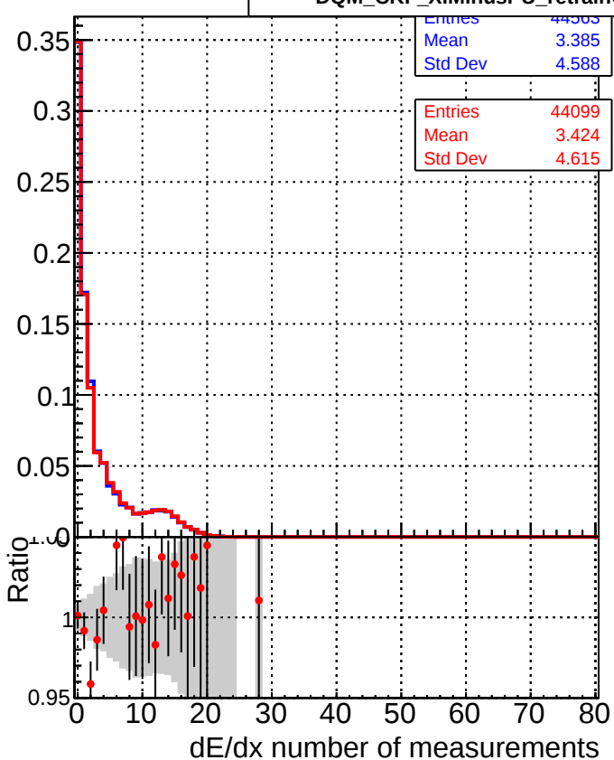
■ DQM_CKF_XiMinusPU_base ● DQM_CKF_XiMinusPU_retrainOldFiles125_v2_prelimWPM_epoch4
