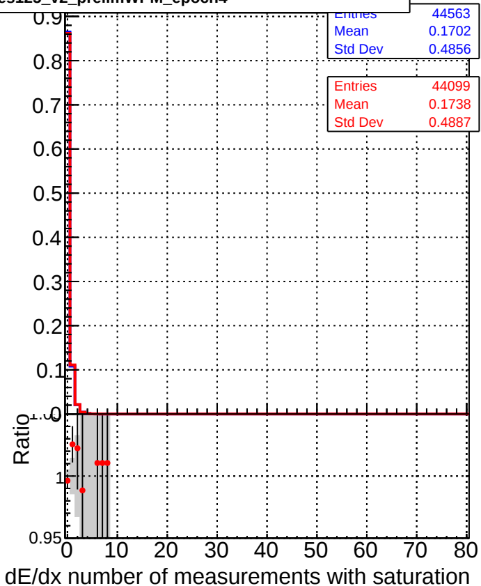
■ DQM_CKF_XiMinusPU_base ● DQM_CKF_XiMinusPU_retrainOldFiles125_v2_prelimWPM_epoch4
