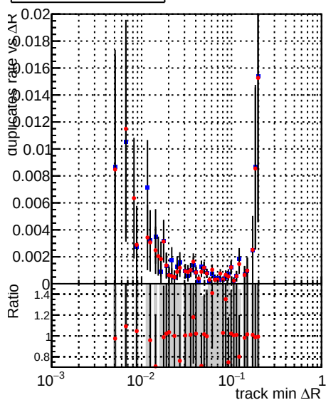
■ DQM_CKF_XiMinusPU_base ● DQM_CKF_XiMinusPU_retrainOldFiles125_v2_prelimWPM_epoch4
