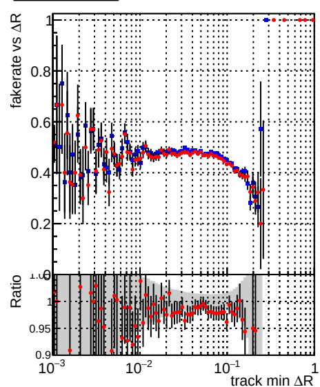
■ DQM_CKF_XiMinusPU_base ● DQM_CKF_XiMinusPU_retrainOldFiles125_v2_prelimWPM_epoch4
