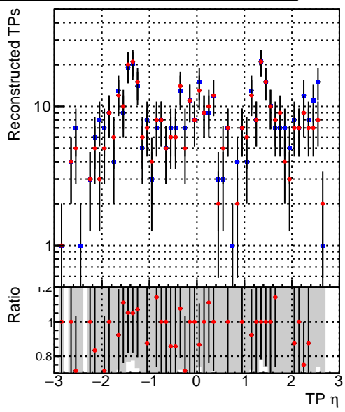
—●— DQM_CKF_XiMinusPU_base —●— DQM_CKF_XiMinusPU_retrainOldFiles125_v2_prelimWPM_epoch3
