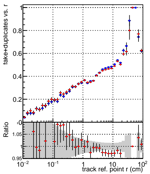
—●— DQM_CKF_XiMinusPU_base —●— DQM_CKF_XiMinusPU_retrainOldFiles125_v2_prelimWPM_epoch3
