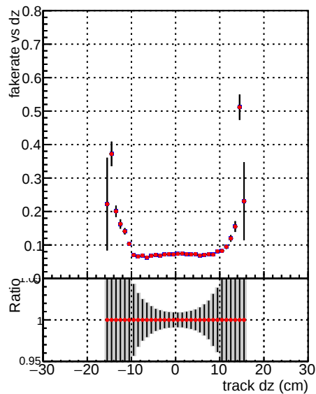
— DQM CKF XiMinusPU_base — DQM CKF XiMinusPU_retrainOldFiles125_v2_prelimWPM_epoch3
