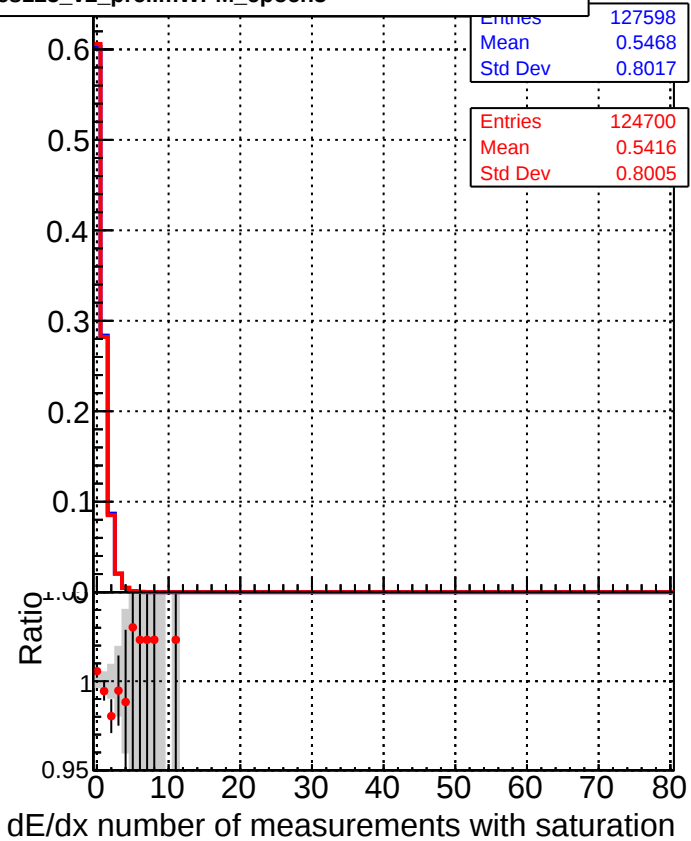
—■— DQM_CKF_XiMinusPU_base —●— DQM_CKF_XiMinusPU_retrainOldFiles125_v2_prelimWPM_epoch3
