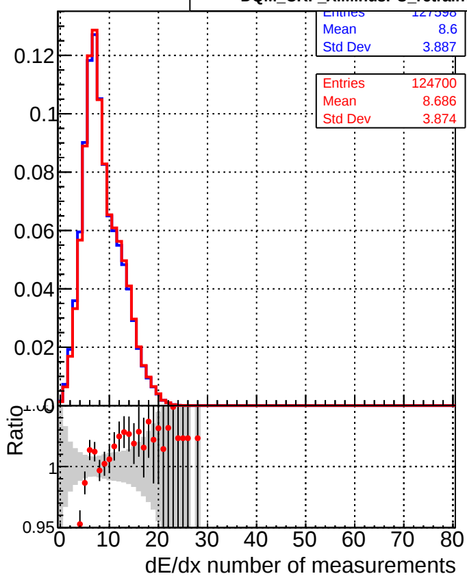
—■— DQM_CKF_XiMinusPU_base —●— DQM_CKF_XiMinusPU_retrainOldFiles125_v2_prelimWPM_epoch3
