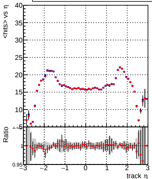
mean hits — DQM_CKF_XiMinusPU_base — DQM_CKF_XiMinusPU_retrainOldFiles125_v2_prelimWPM_epoch3
