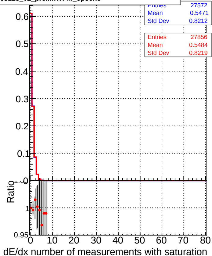
—■— DQM_CKF_XiMinusPU_base —●— DQM_CKF_XiMinusPU_retrainOldFiles125_v2_prelimWPM_epoch3
