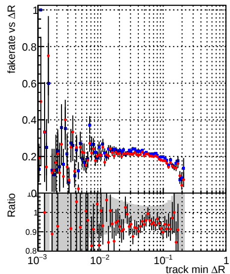
■ DQM_CKF_XiMinusPU_base ● DQM_CKF_XiMinusPU_retrainOldFiles125_v2_prelimWPM_epoch3
