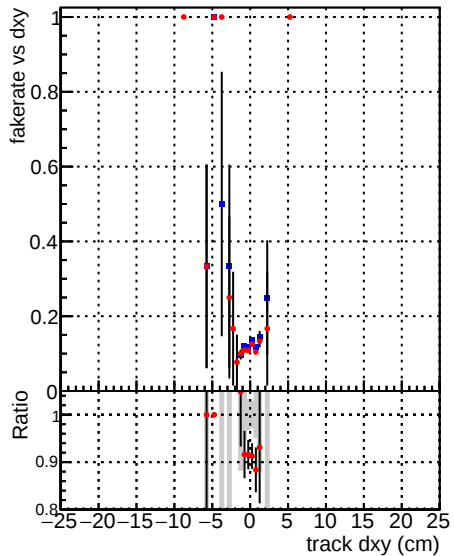
—●— DQM_CKF_XiMinusPU_base —●— DQM_CKF_XiMinusPU_retrainOldFiles125_v2_prelimWPM_epoch3
