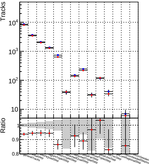
■ DQM_CKF_XiMinusPU_base
