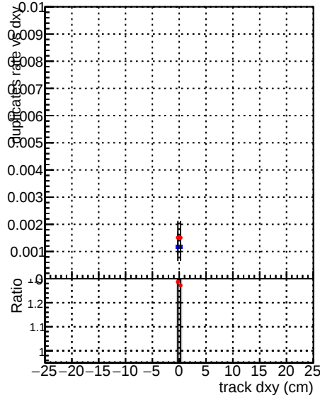
—●— DQM_CKF_XiMinusPU_base —●— DQM_CKF_XiMinusPU_retrainOldFiles125_v2_prelimWPM_epoch3
