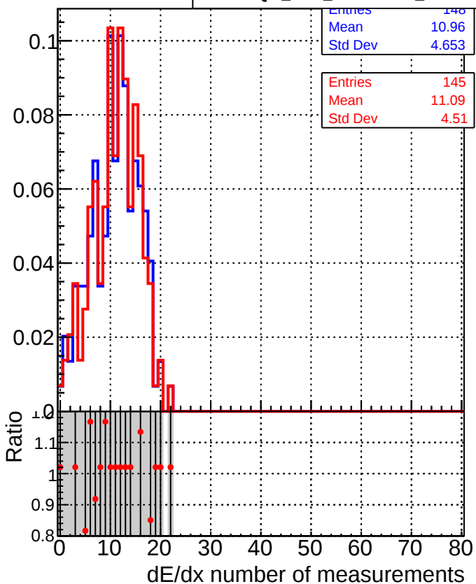
■ DQM_CKF_XiMinusPU_base ● DQM_CKF_XiMinusPU_retrainOldFiles125_v2_prelimWPM_epoch3
