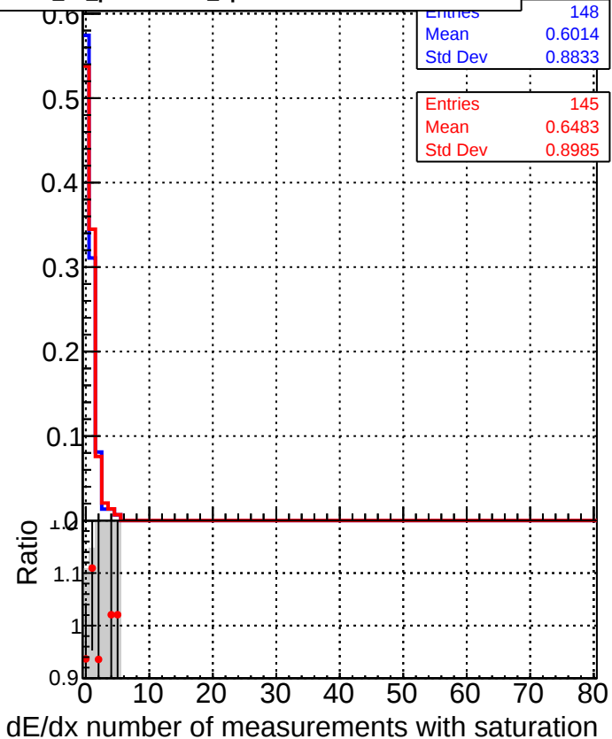
■ DQM_CKF_XiMinusPU_base ● DQM_CKF_XiMinusPU_retrainOldFiles125_v2_prelimWPM_epoch3
