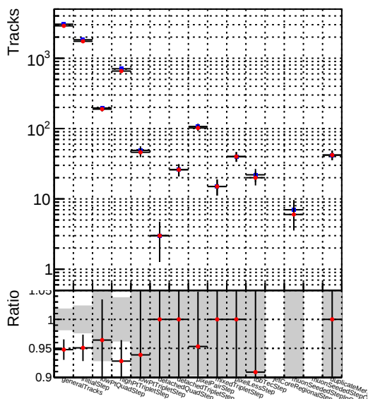
■ DQM_CKF_XiMinusPU_base
