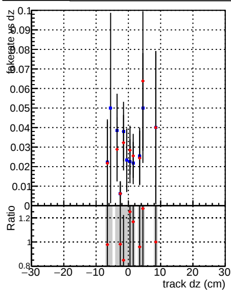
—•— DQM_CKF_XiMinusPU_base —•— DQM_CKF_XiMinusPU_retrainOldFiles125_v2_prelimWPM_epoch3
