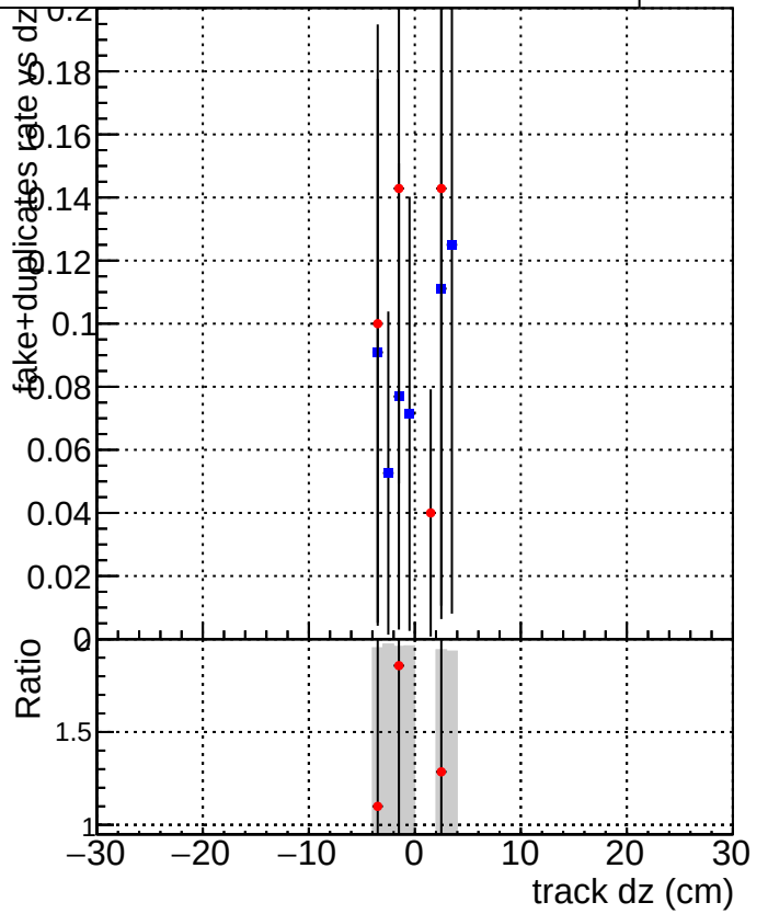
DQM_CKF_XiMinusPU_base DQM_CKF_XiMinusPU_retrainOldFiles125_v2_prelimWPM_epoch3
