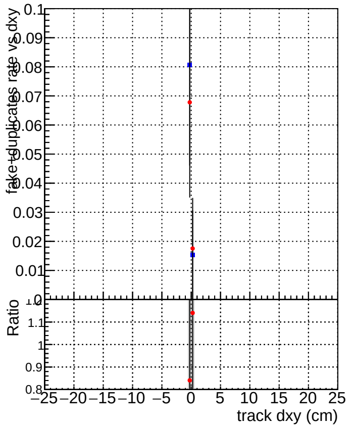
DQM_CKF_XiMinusPU_base DQM_CKF_XiMinusPU_retrainOldFiles125_v2_prelimWPM_epoch3
