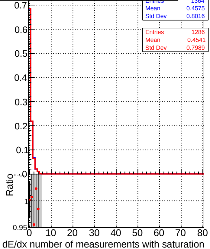
DQM_CKF_XiMinusPU_base DQM_CKF_XiMinusPU_retrainOldFiles125_v2_prelimWPM_epoch3
