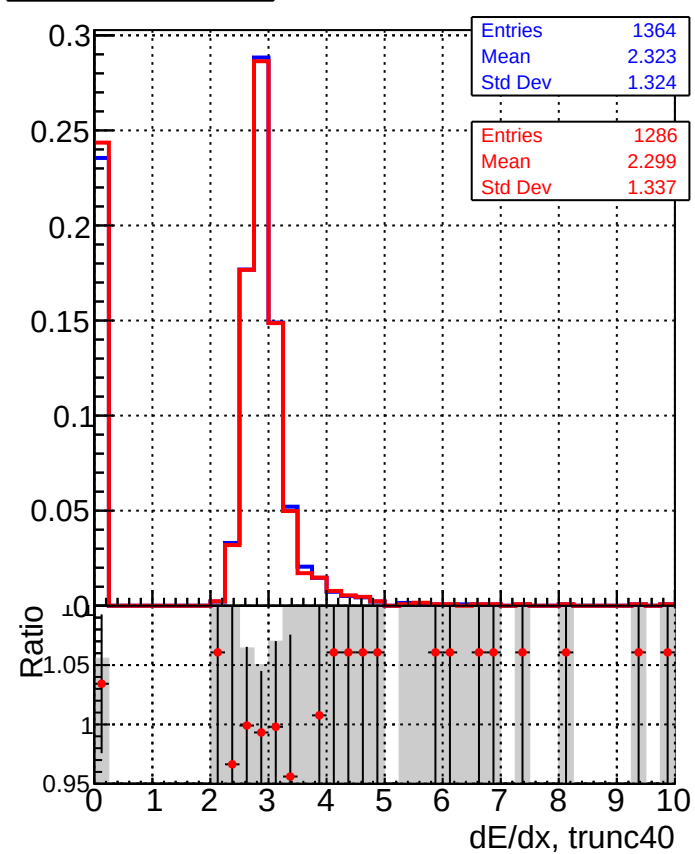
DQM_CKF_XiMinusPU_base DQM_CKF_XiMinusPU_retrainOldFiles125_v2_prelimWPM_epoch3
