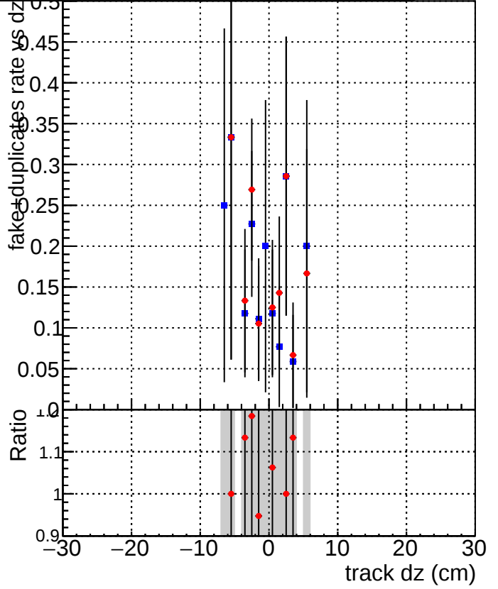
DQM_CKF_XiMinusPU_base DQM_CKF_XiMinusPU_retrainOldFiles125_v2_prelimWPM_epoch3
