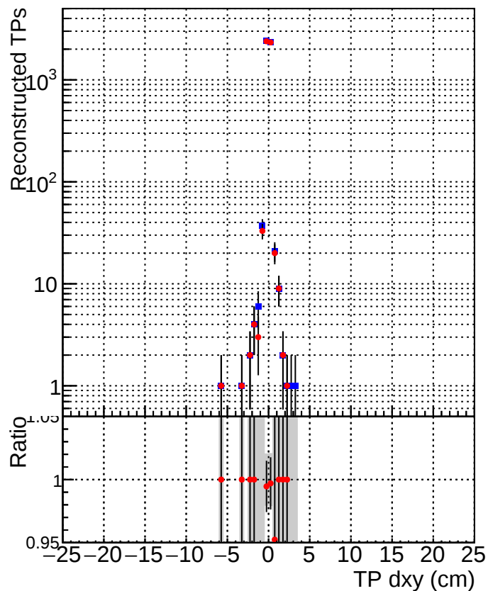
DQM_CKF_XiMinusPU_base DQM_CKF_XiMinusPU_retrainOldFiles125_v2_prelimWPM_epoch3
