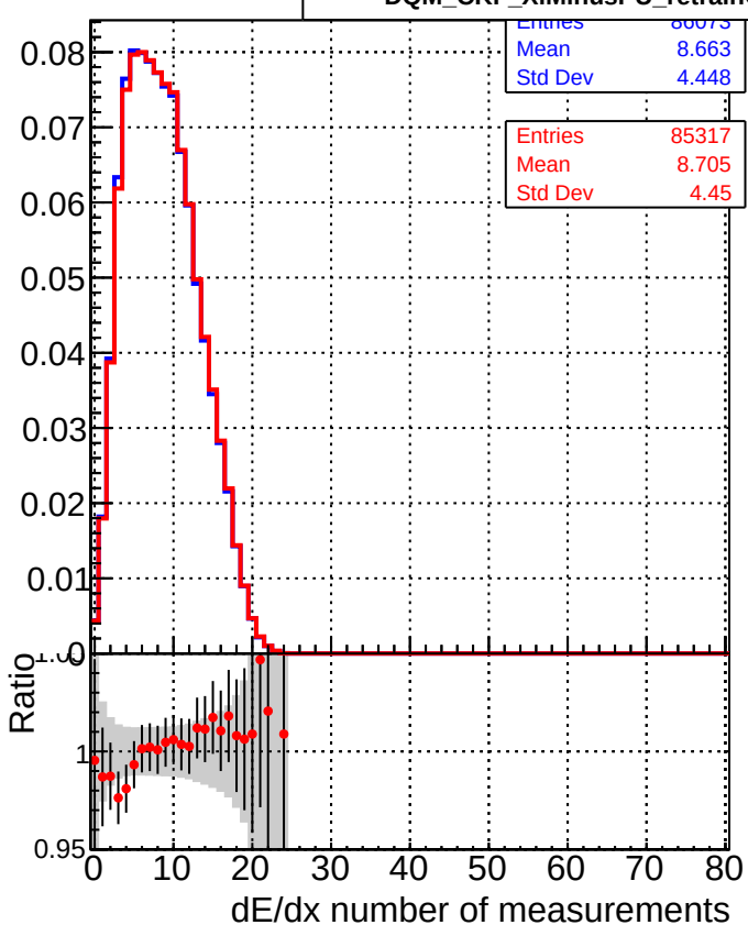
DQM_CKF_XiMinusPU_base DQM_CKF_XiMinusPU_retrainOldFiles125_v2_prelimWPM_epoch3
