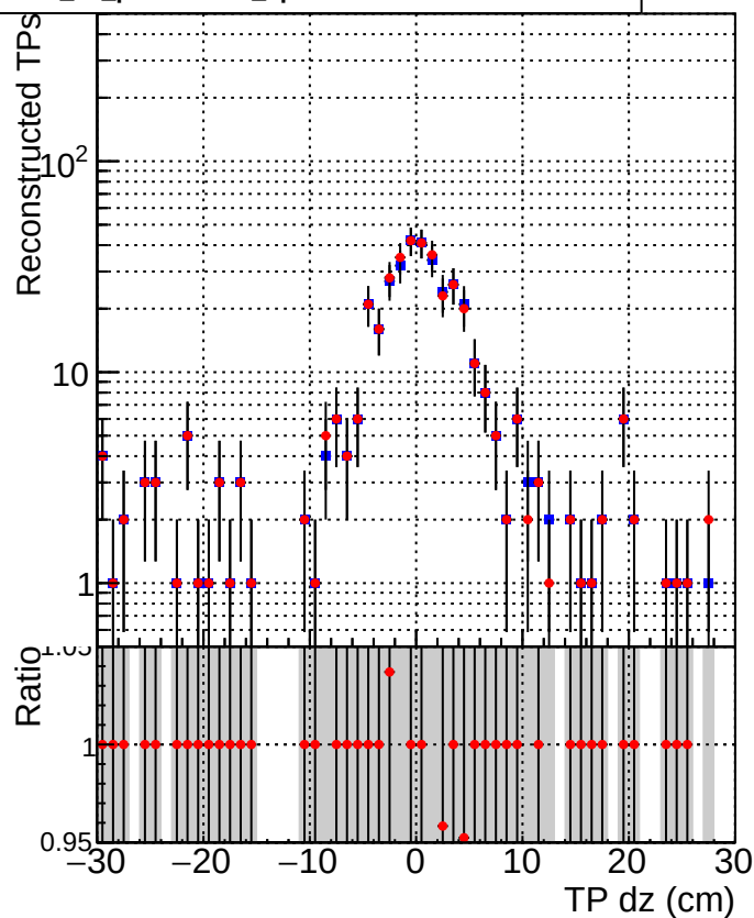
■ DQM_CKF_XiMinusPU_base ● DQM_CKF_XiMinusPU_retrainOldFiles125_v2_prelimWPM_epoch2
