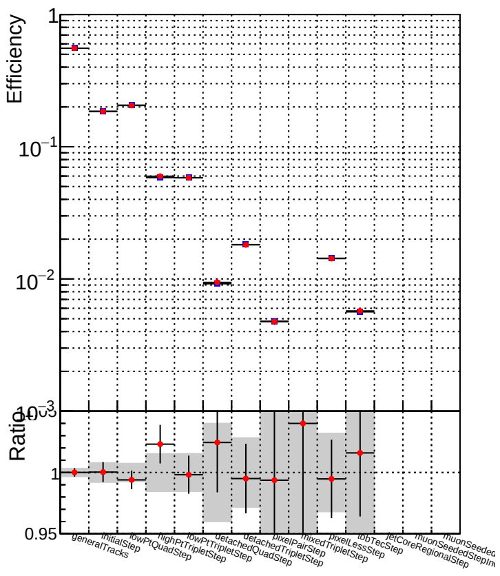
DQM_CKF_XiMinusPU_base DQM_CKF_XiMinusPU_retrainOldFiles125_v2_prelimWPM_epoch2
