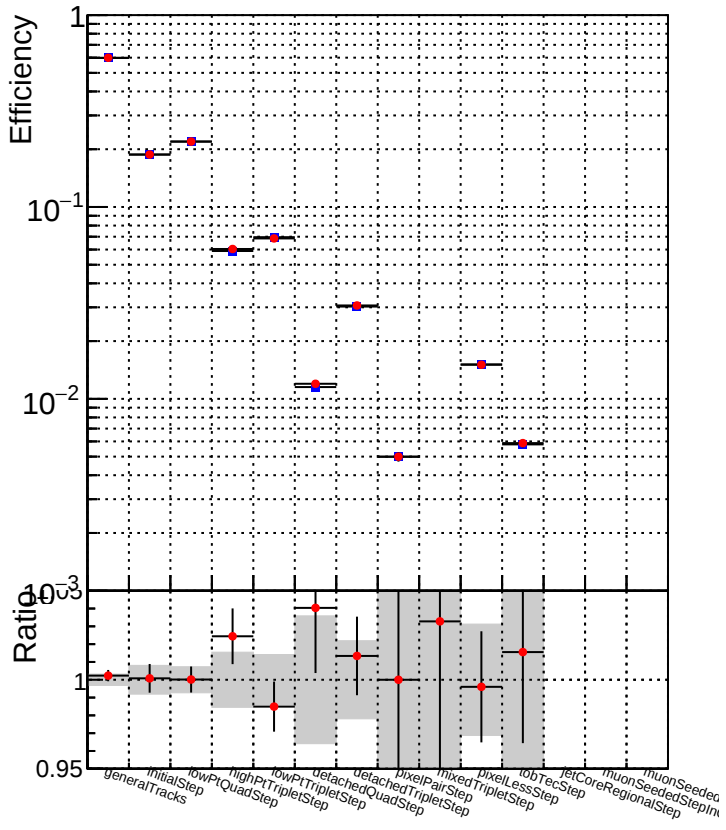
DQM_CKF_XiMinusPU_base DQM_CKF_XiMinusPU_retrainOldFiles125_v2_prelimWPM_epoch2
