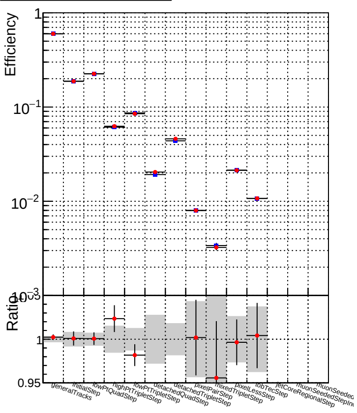
DQM_CKF_XiMinusPU_base DQM_CKF_XiMinusPU_retrainOldFiles125_v2_prelimWPM_epoch2
