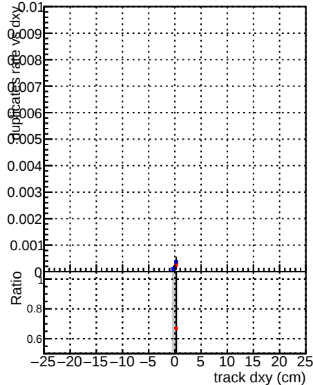
—●— DQM_CKF_XiMinusPU_base —●— DQM_CKF_XiMinusPU_retrainOldFiles125_v2_prelimWPM_epoch2
