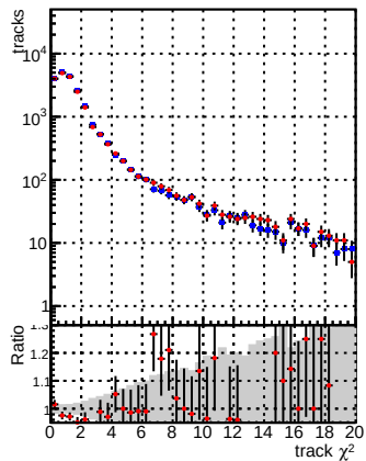
—●— DQM_CKF_XiMinusPU_base —●— DQM_CKF_XiMinusPU_retrainOldFiles125_v2_prelimWPM_epoch2
