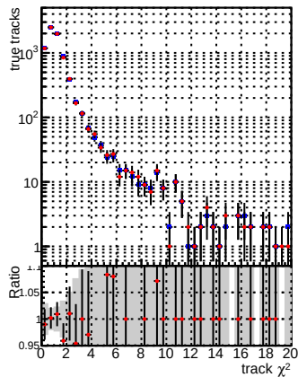
—●— DQM_CKF_XiMinusPU_base —●— DQM_CKF_XiMinusPU_retrainOldFiles125_v2_prelimWPM_epoch2
