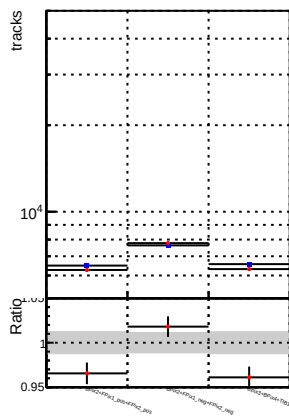
—●— DQM_CKF_XiMinusPU_base —●— DQM_CKF_XiMinusPU_retrainOldFiles125_v2_prelimWPM_epoch2
