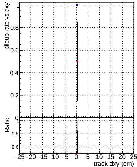
DQM CKF_XiMinusPU_retrainOldFiles125_v2_prelimWPM_epoch2
