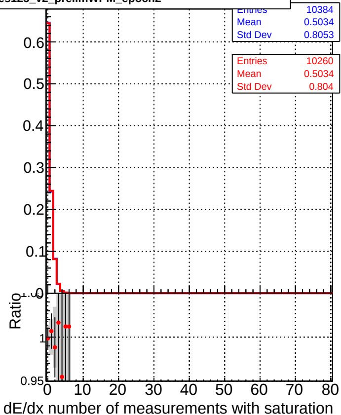
■ DQM_CKF_XiMinusPU_base ● DQM_CKF_XiMinusPU_retrainOldFiles125_v2_prelimWPM_epoch2
