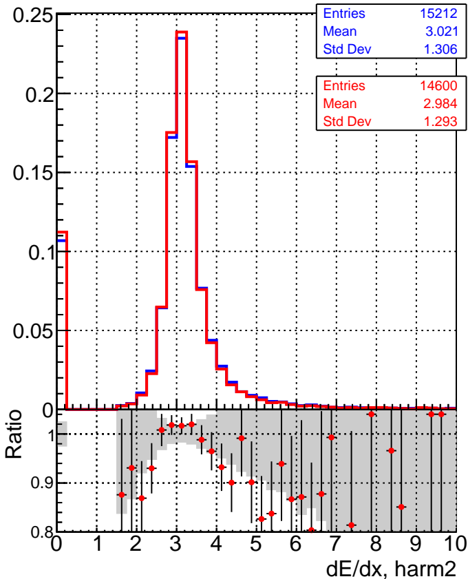
—■— DQM_CKF_XiMinusPU_base
