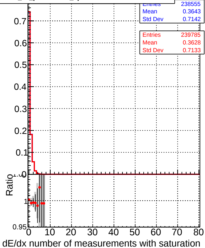
DQM_CKF_XiMinusPU_base DQM_CKF_XiMinusPU_retrainOldFiles125_v2_prelimWPM_epoch2
