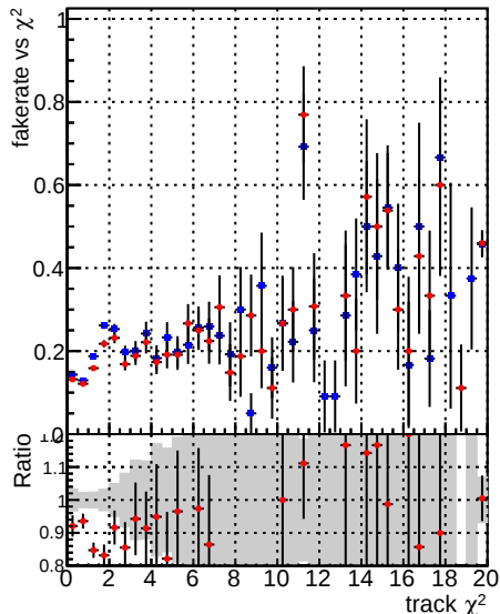
Fake rate vs. —◆— DQM CKF XiMinusPU_base —●— DQM CKF XiMinusPU_retrainOldFiles125_v2_prelimWPM_epoch2
