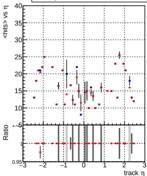
— DQM_CKF_XiMinusPU_base — DQM_CKF_XiMinusPU_retrainOldFiles125_v2_prelimWPM_epoch2
