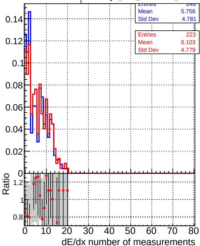
■ DQM_CKF_XiMinusPU_base ● DQM_CKF_XiMinusPU_retrainOldFiles125_v2_prelimWPM_epoch2
