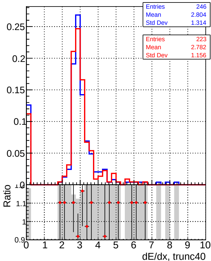
■ DQM_CKF_XiMinusPU_base ● DQM_CKF_XiMinusPU_retrainOldFiles125_v2_prelimWPM_epoch2
