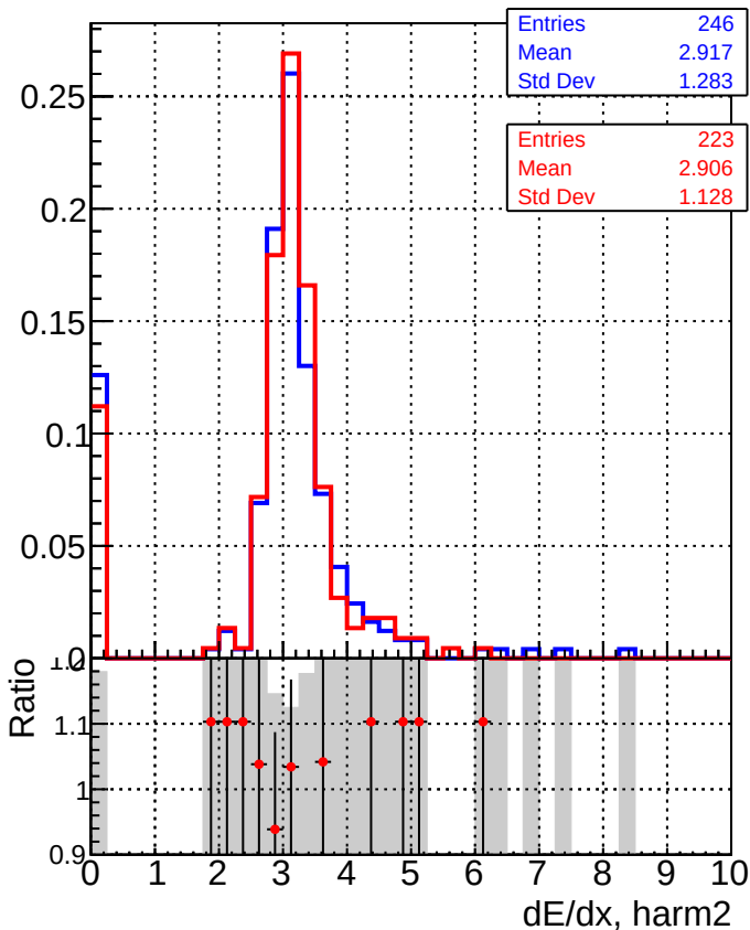
■ DQM_CKF_XiMinusPU_base ● DQM_CKF_XiMinusPU_retrainOldFiles125_v2_prelimWPM_epoch2
