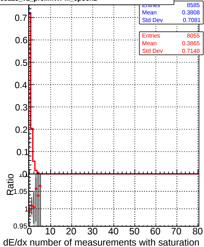
■ DQM_CKF_XiMinusPU_base ● DQM_CKF_XiMinusPU_retrainOldFiles125_v2_prelimWPM_epoch2
