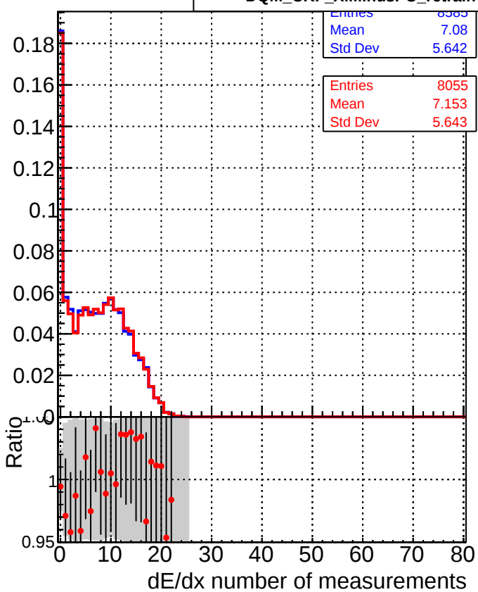
■ DQM_CKF_XiMinusPU_base ● DQM_CKF_XiMinusPU_retrainOldFiles125_v2_prelimWPM_epoch2
