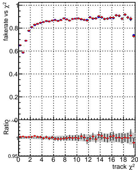
—• DQM_CKF_XiMinusPU_base —• DQM_CKF_XiMinusPU_retrainOldFiles125_v2_prelimWPM_epoch2
