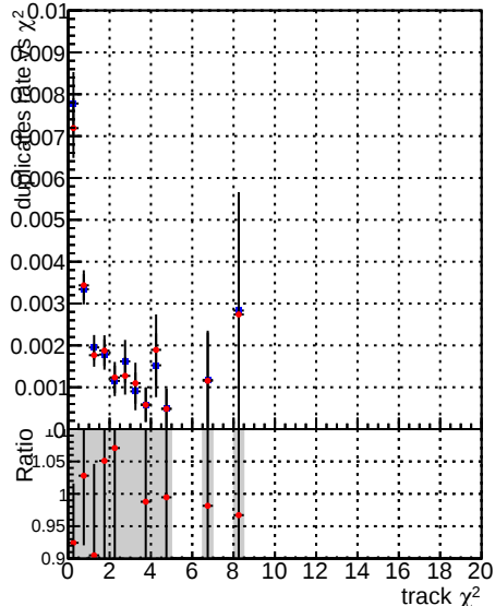
—●— DQM_CKF_XiMinusPU_base —●— DQM_CKF_XiMinusPU_retrainOldFiles125_v2_prelimWPM_epoch2
