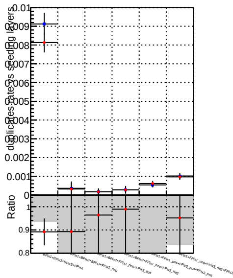
—●— DQM_CKF_XiMinusPU_base —●— DQM_CKF_XiMinusPU_retrainOldFiles125_v2_prelimWPM_epoch2
