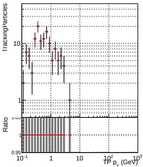
— DQM_CKF_XiMinusPU_base — DQM_CKF_XiMinusPU_retrainOldFiles125_v2_prelimWPM_epoch2
