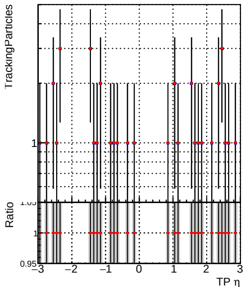
— DQM_CKF_XiMinusPU_base — DQM_CKF_XiMinusPU_retrainOldFiles125_v2_prelimWPM_epoch2
