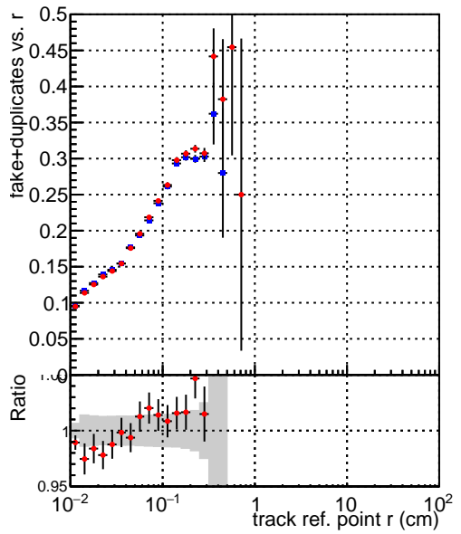
—●— DQM_CKF_XiMinusPU_base —●— DQM_CKF_XiMinusPU_retrainOldFiles125_v2_prelimWPM_epoch2
